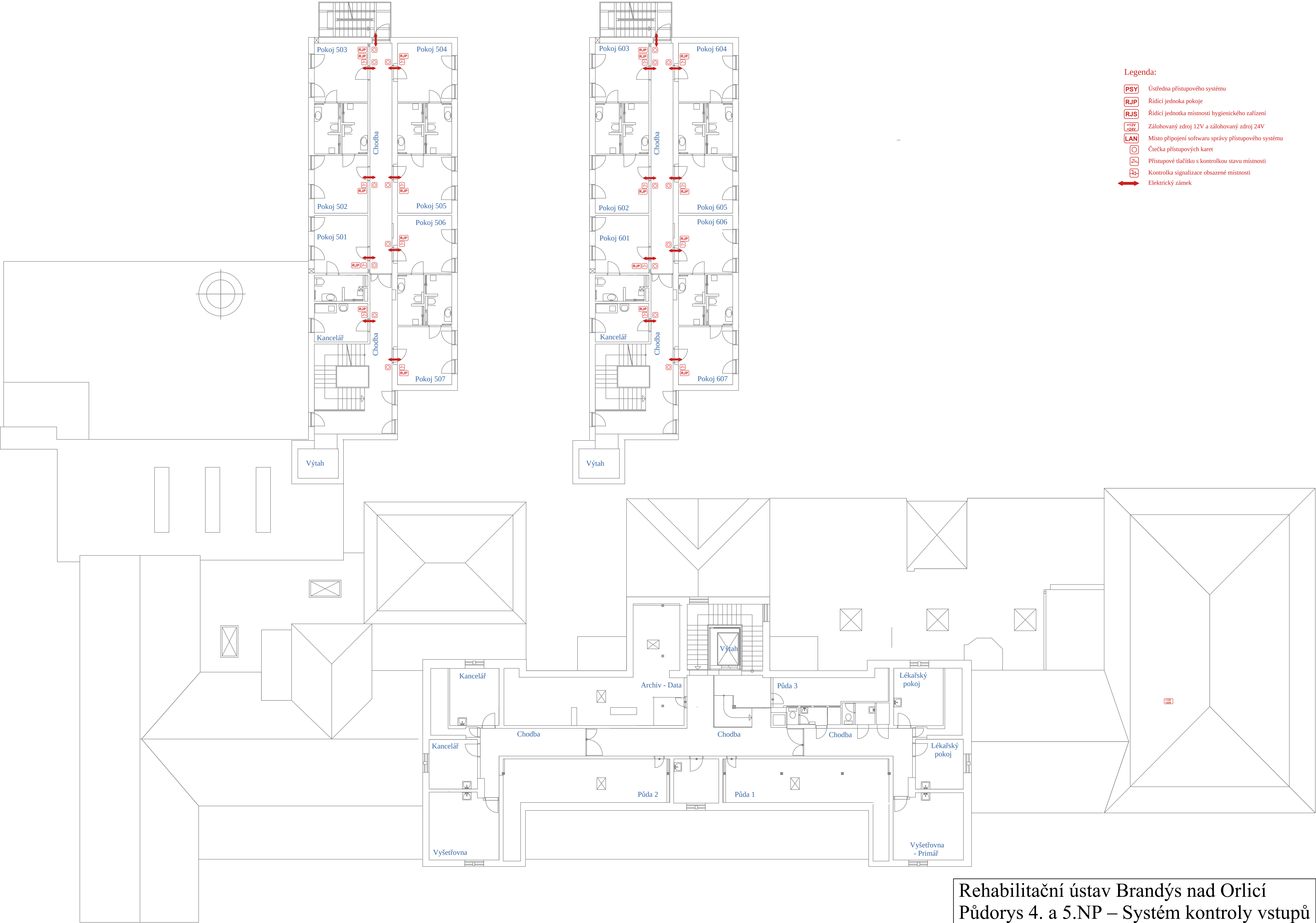
Půdorys 4.NP
